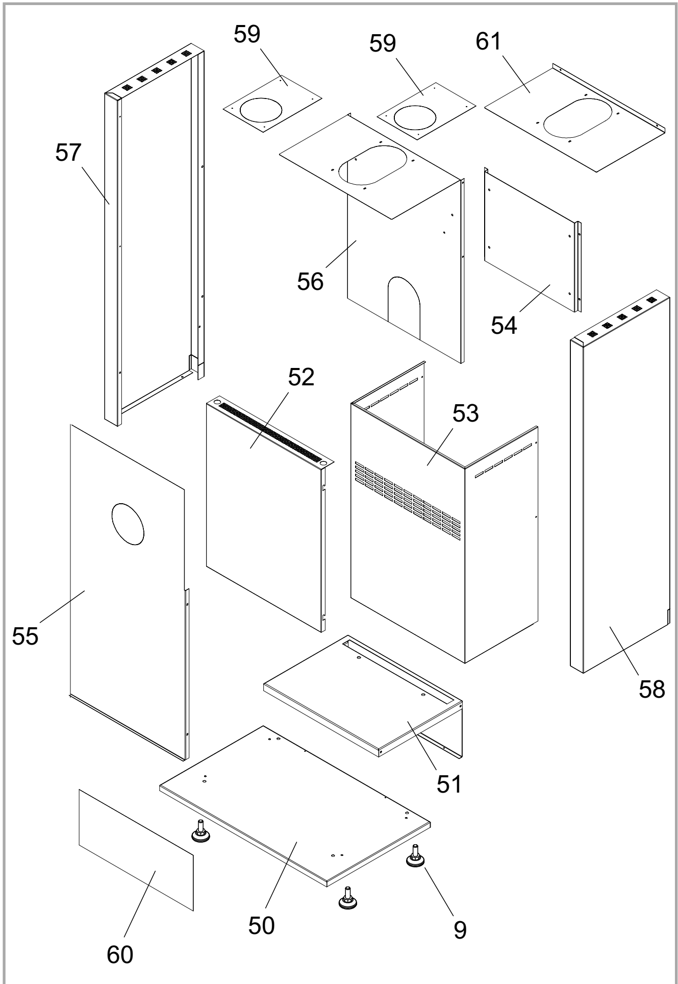
Figure 12 - Vue éclatée de l'appareil 134 10 24 Y
