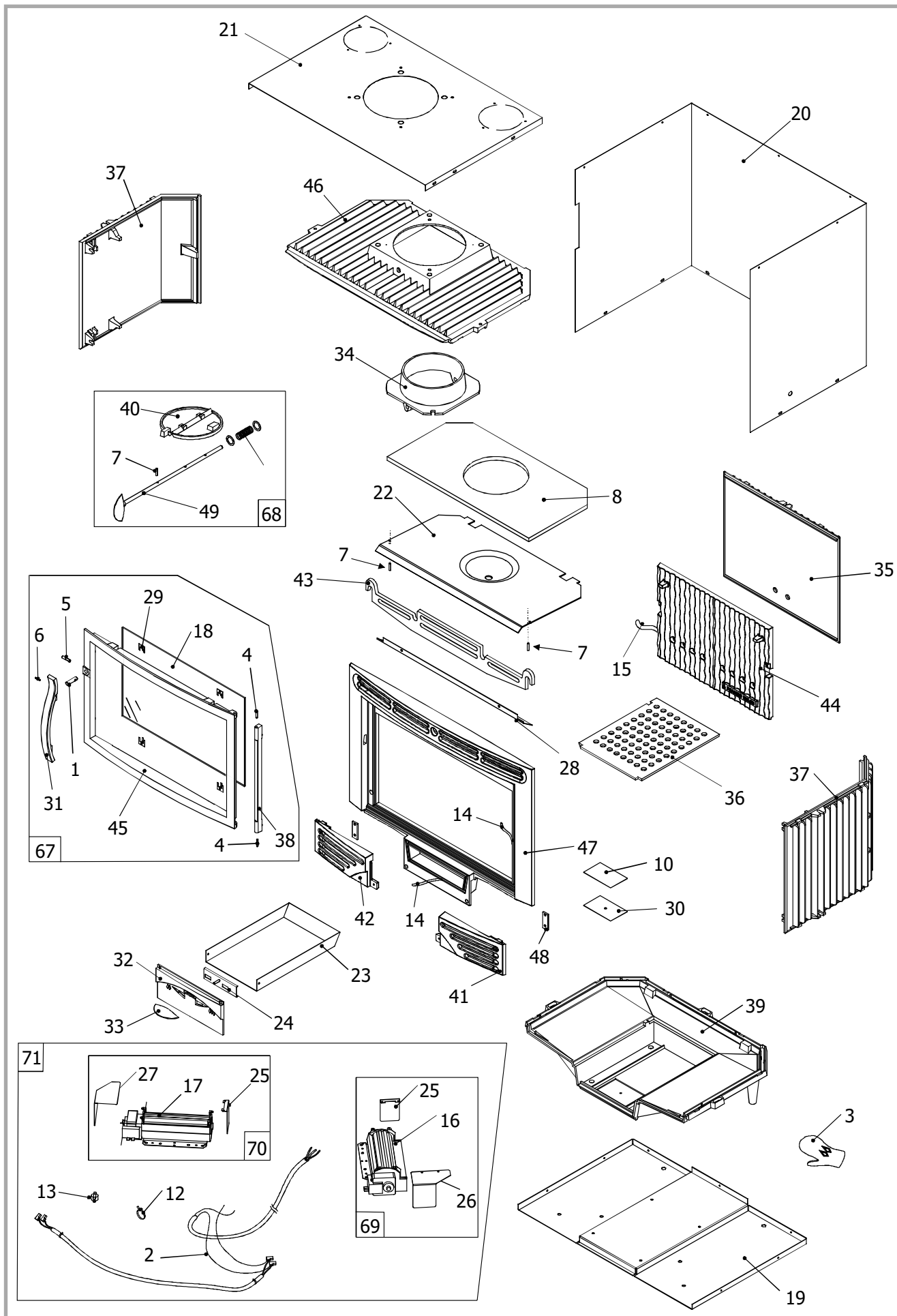
Figure 11 - Vue éclatée de l'appareil 134 10 24 Y
