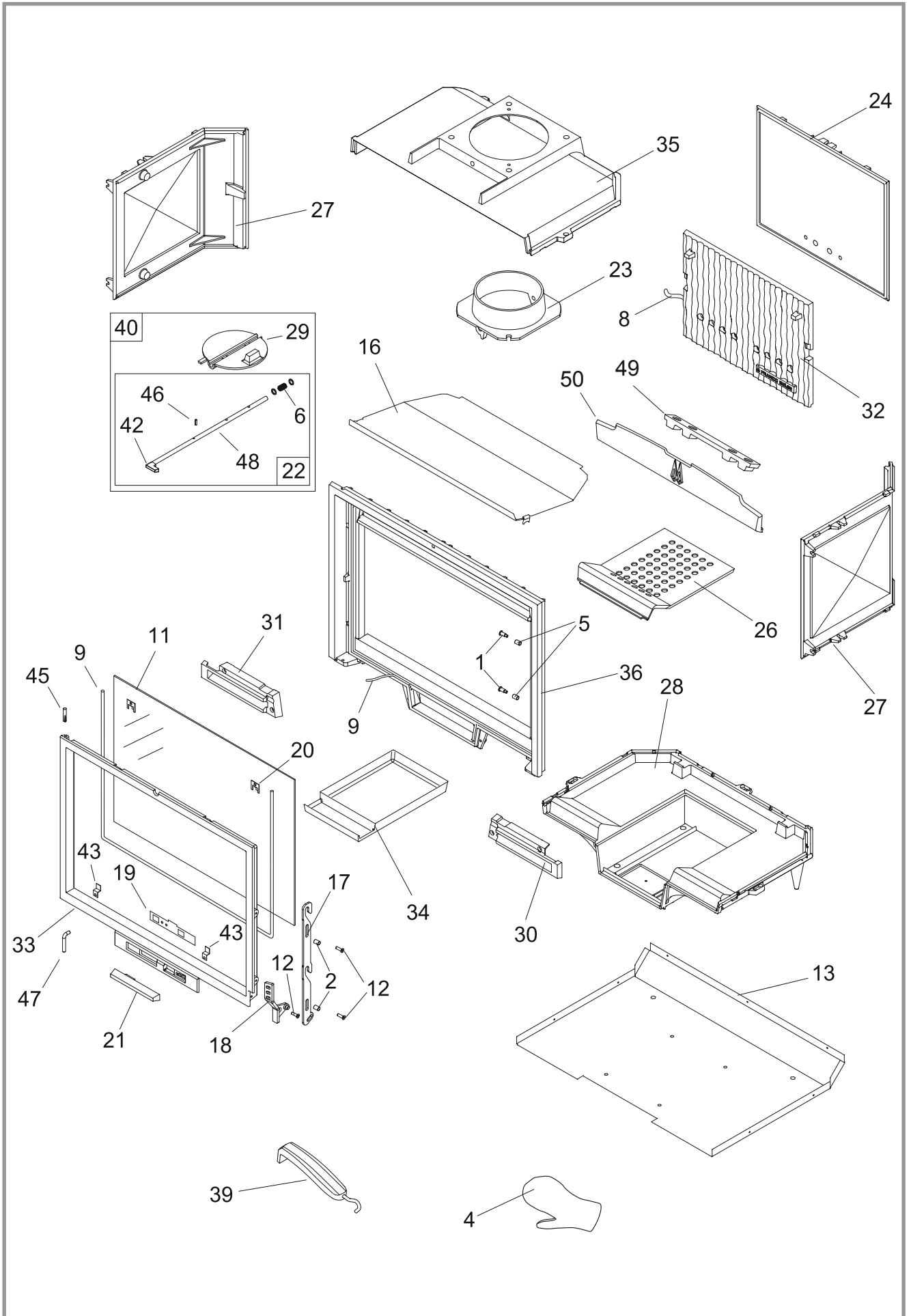
Figure 14 - Vue éclaté de l'appareil
